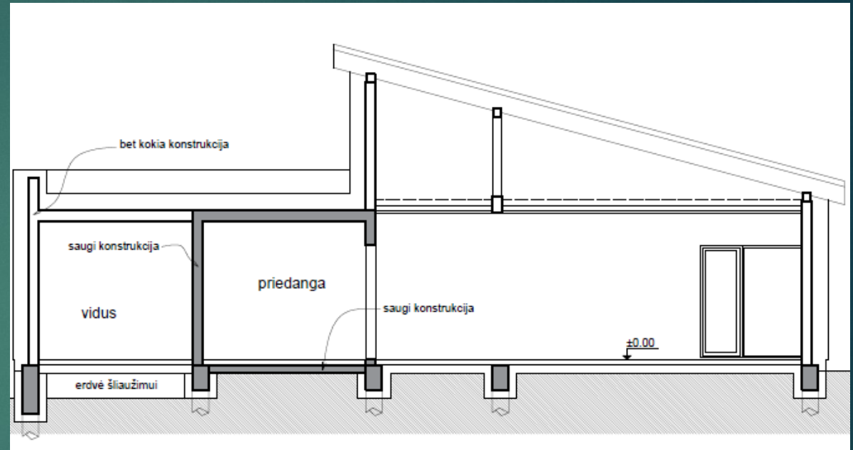
Pav. PSP vieta individualiame name (pjūvis)
