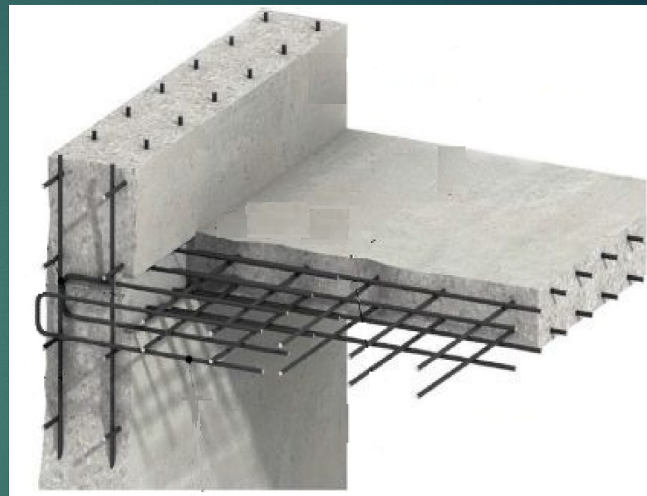
Pav. Betoninės sienos jungtis su perdanga
