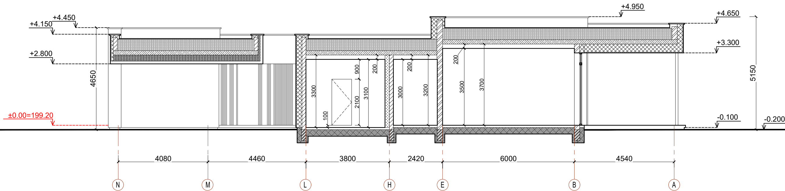
PJŪVIS 1-1
