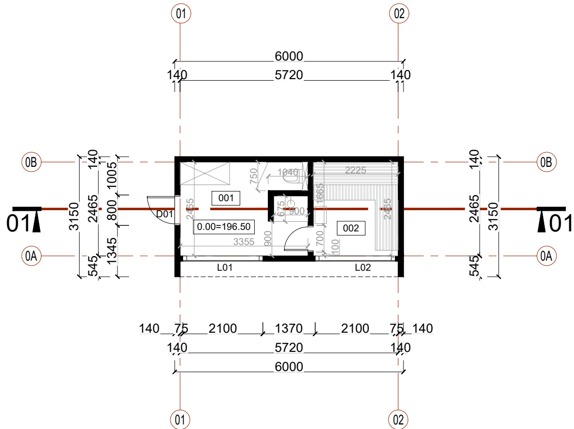
PIRMO AUKŠTO PLANAS M 1:100
