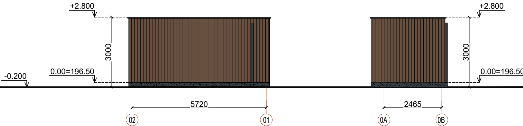
FASADAI TAP AŠIŲ 02-01, 0A-0B M 1:100
