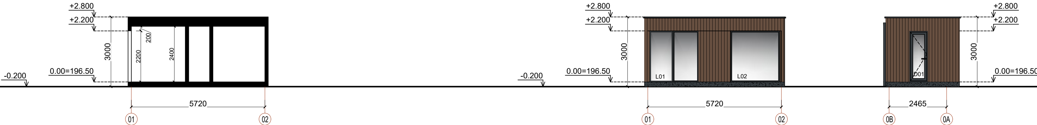
FASADAI TAP AŠIŲ 01-02, 0B-0A M 1:100
