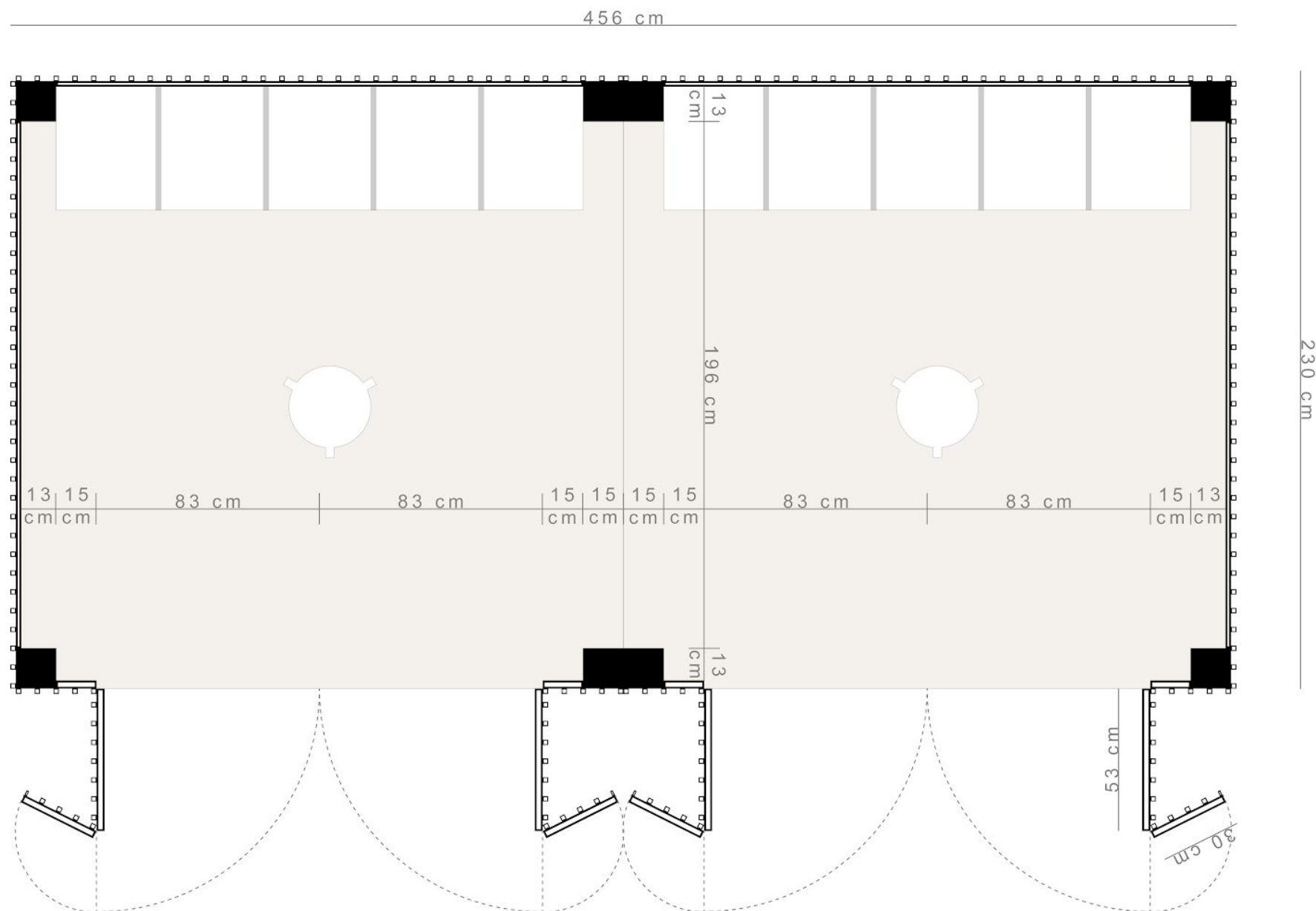
Tipinis dvigubo paviljono planas
