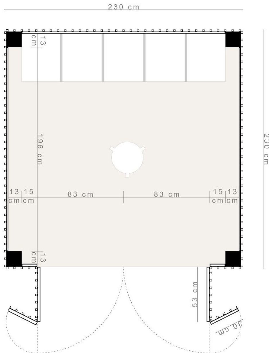
Tipinis paviljono planas
