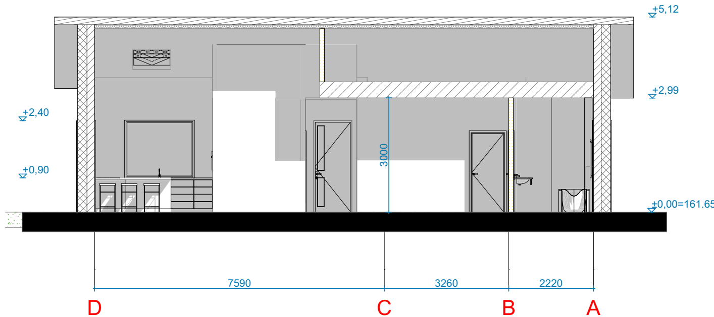
ARCHITEKTŪRINIS PJŪVIS 1-1
