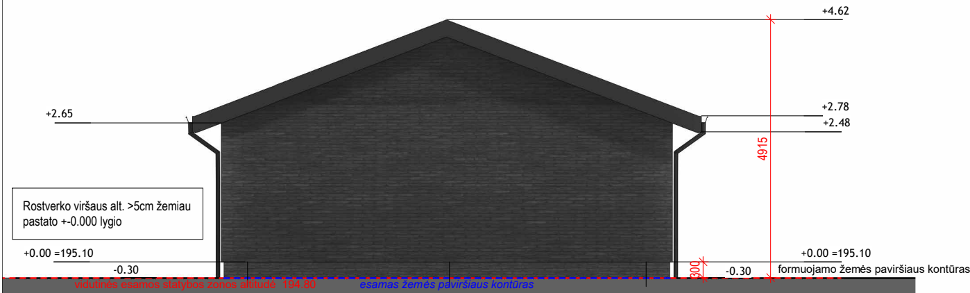
Fasadas 3-1, M1:100
