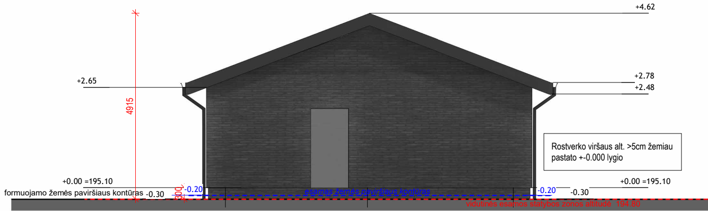
Fasadas 1-3, M1:100
