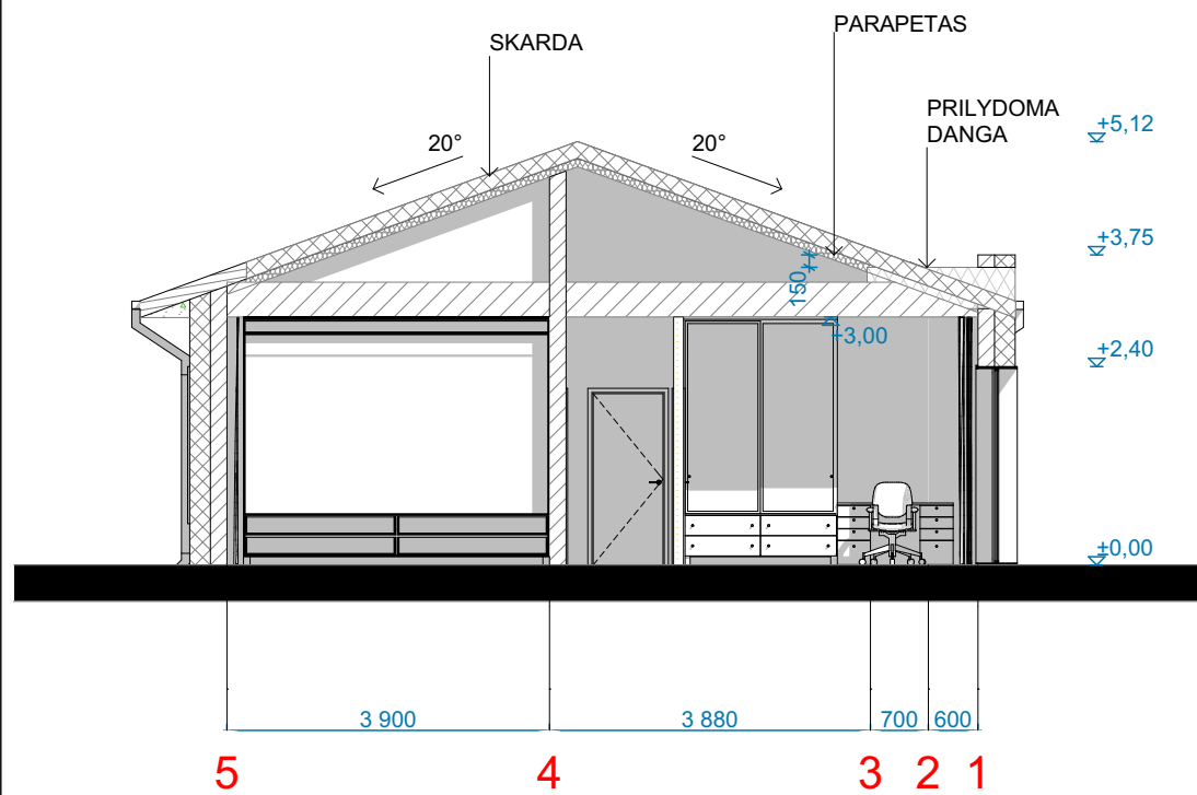
ARCHITEKTŪRINIS PJŪVIS 3-3
