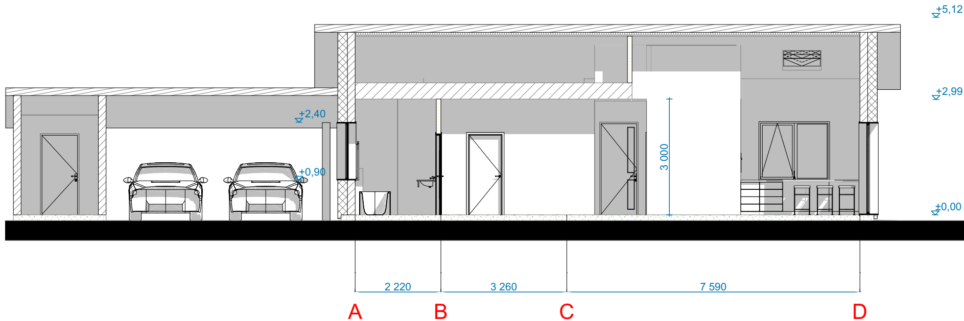
ARCHITEKTŪRINIS PJŪVIS 1-1
