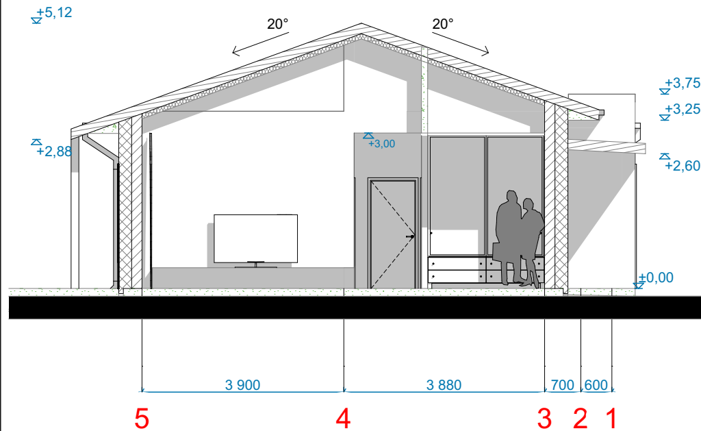
ARCHITEKTŪRINIS PJŪVIS 2-2
